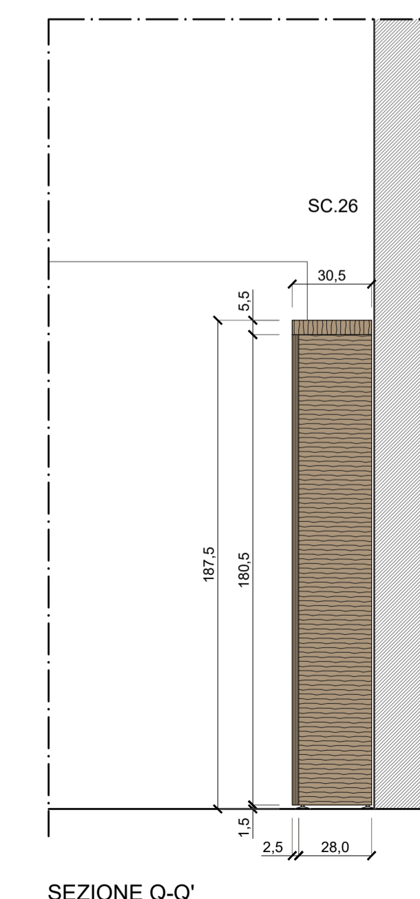
SEZIONE Q-Q'
