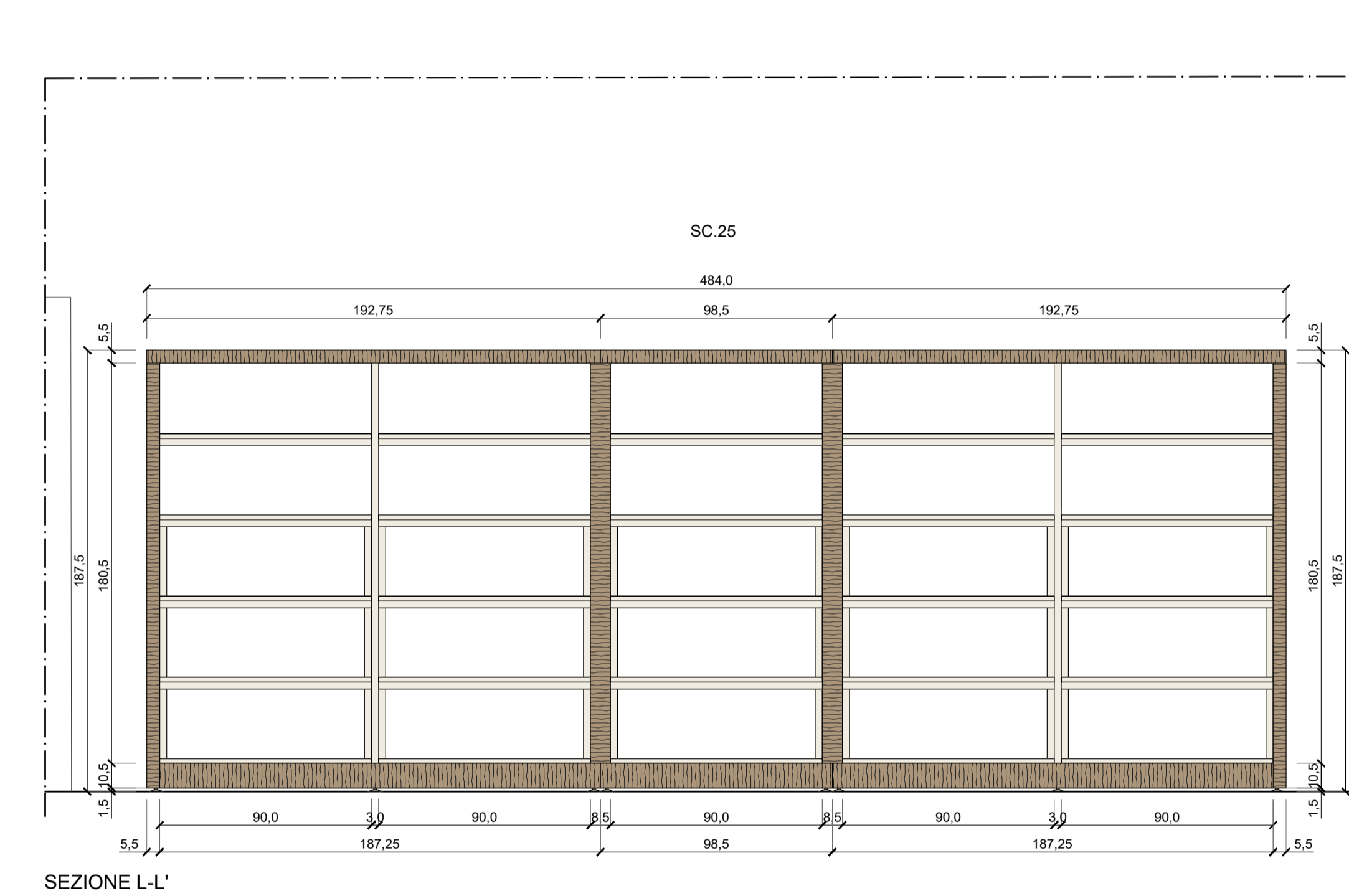
SEZIONE L-L'
