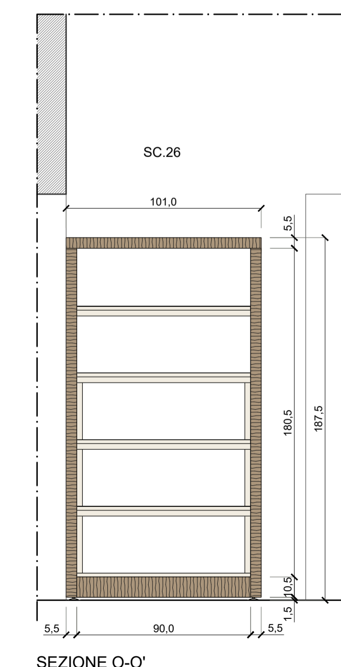
SEZIONE O-O'
