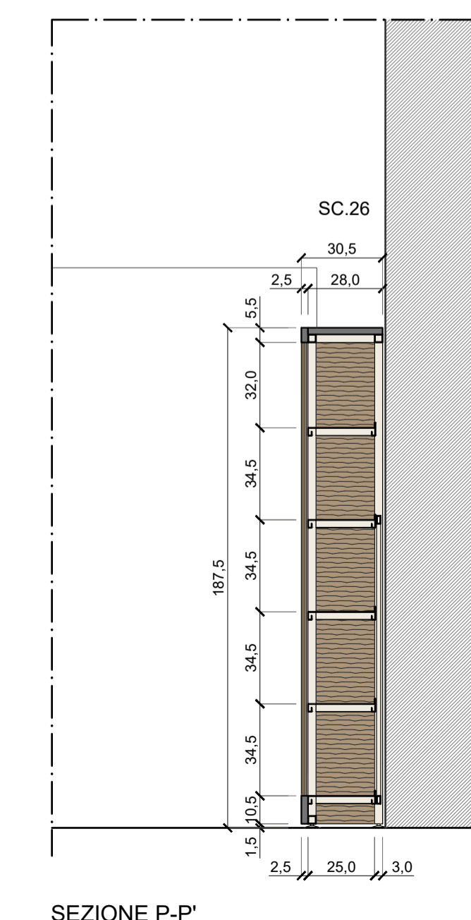
SEZIONE P-P'
