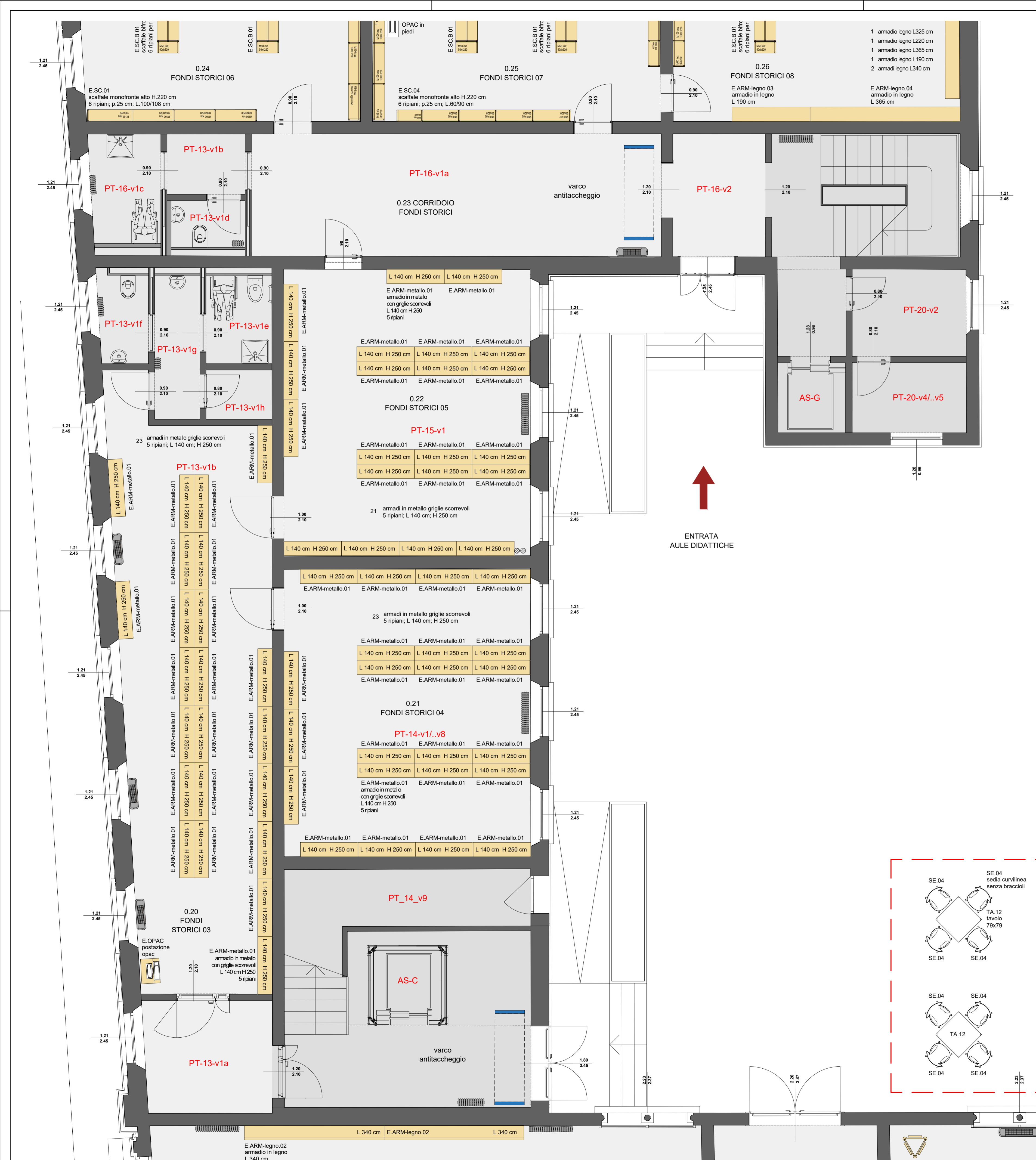
PIANTA ARREDATA PIANO TERRA | ESTRATTO "B" scala 1:50
